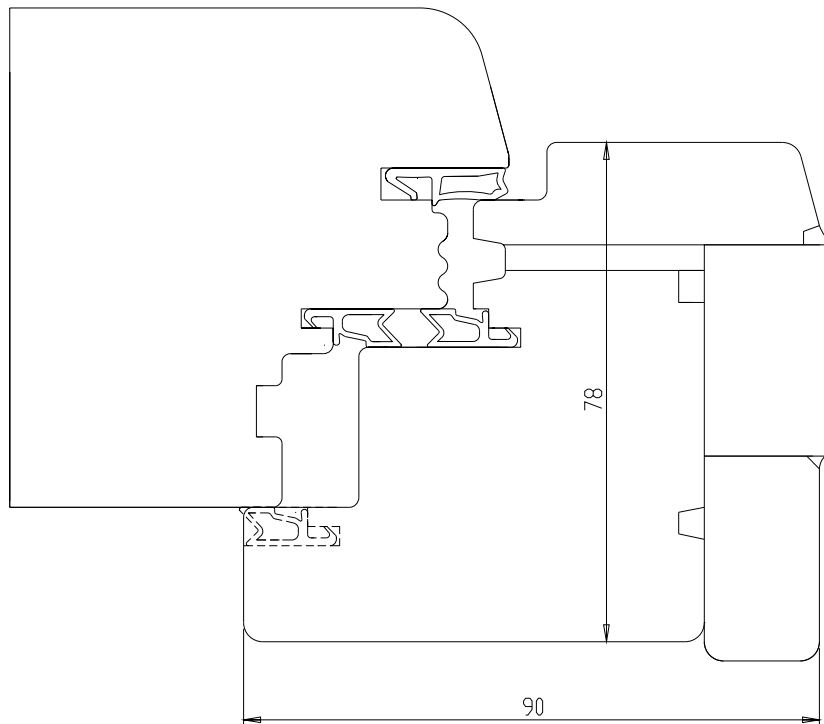
SERIE CLIMATAC PLUS/78 Lateral superior, izquierdo y derecho
